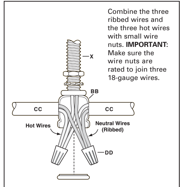
FIG 13. CLUSTER WIRING
